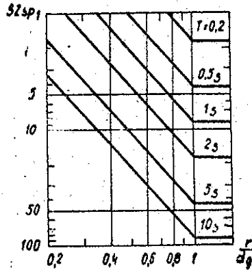
Rys. 2. Spadek zrozumiałości spótgłosek w funkcji r/d dla różnych wartości czasu pogłosu
