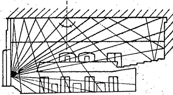
Rys. 1. Analiza graficzna biegu promieni dźwiękowych dla podłużnego przekroju sali. W poprawnie zaprojektowanych pomieszczeniach włązki odbite np. 1-szego odbicia nie powinny się ogniskować
