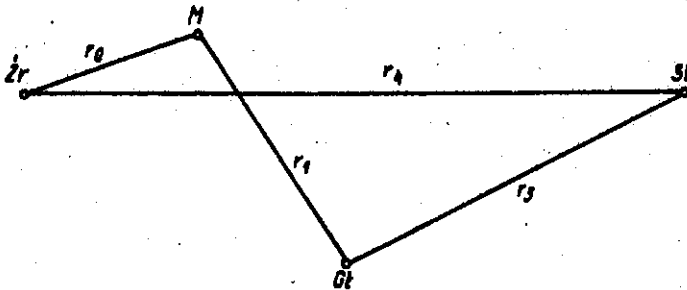
Rys. 6. Rozmieszczenie: źródła naturalnego Z_r , mikrofonu M , głośnika G_{\text{ł}} , słuchacza S_{\text{ł}} , w obszarze nagłośnionym
