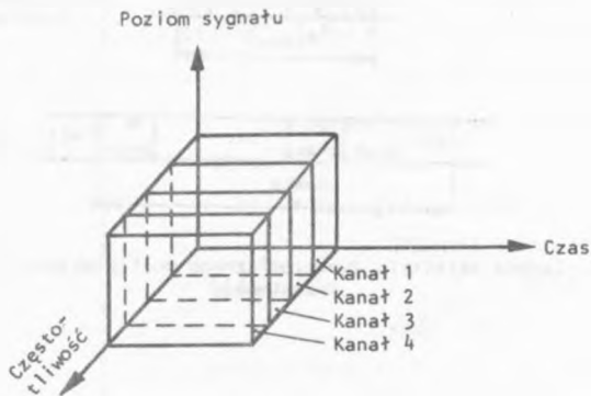
Rys. 1. Zasada wielokrotnienia częstotliwościowego
