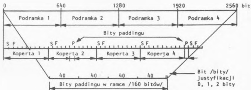
Ramka zwielokrotnienia zgodna z zaleceniem X.51
