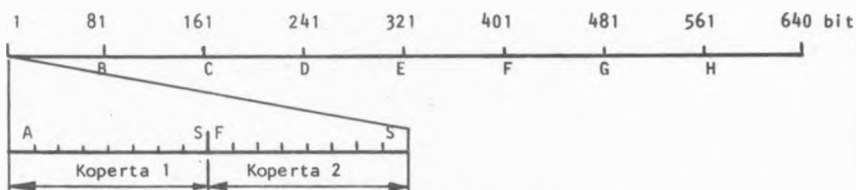
Ramka zwielokrotnienia zgodna z zaleceniem X.50
