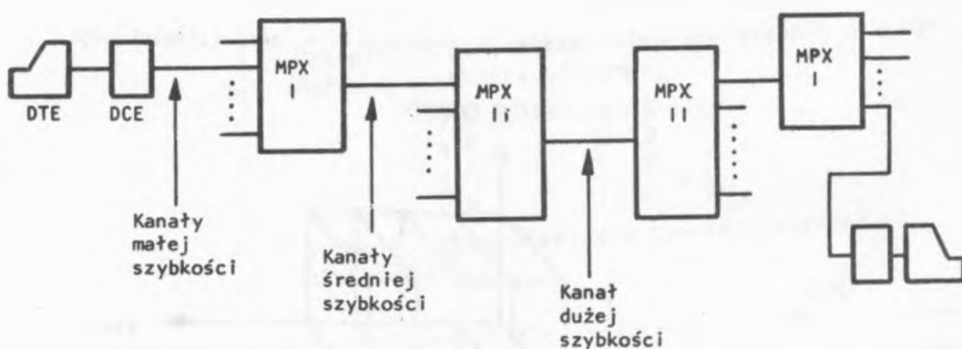
Rys. 4. Wybrany przykład hierarchicznego połączenia multipleksorów w sieci transmisji danych
