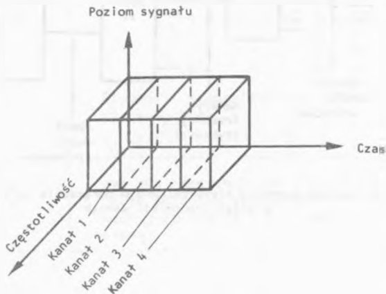
Rys. 2. Zasada wielokrotnienia czasowego
