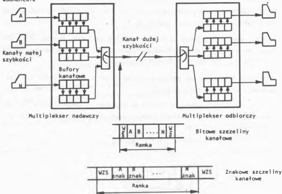
Rys. 3. Zasada działania synchronicznego multipleksera bitowego i znakowego
