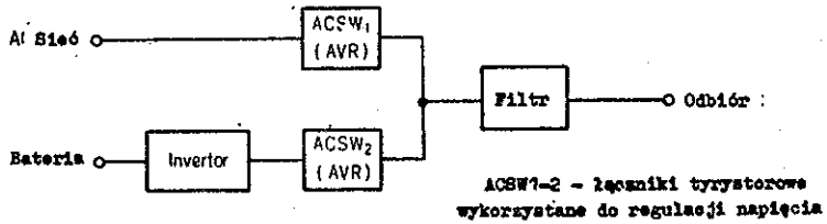
Rys. 3. Różne metody regulacji napięcia
