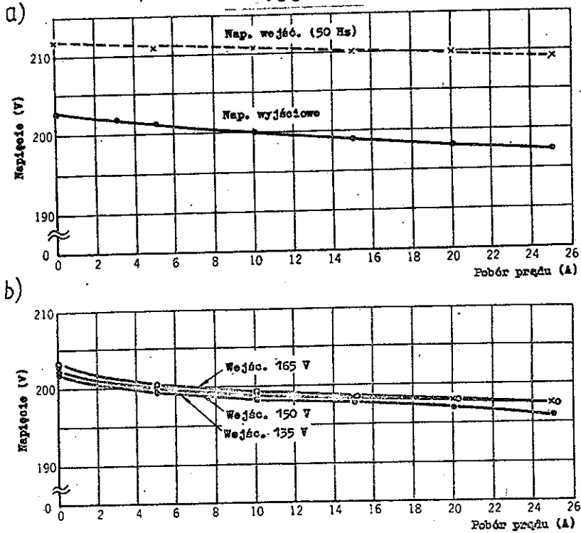
Rys. 5. Charakterystyki napięciowe przy badaniach końcowych: a) podczas zasilania z sieci, b) podczas zasilania z przetwornicy
