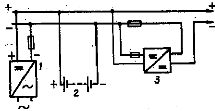
Rys. 3. Schemat blokowy systemu z przetwornicą dodatkową
