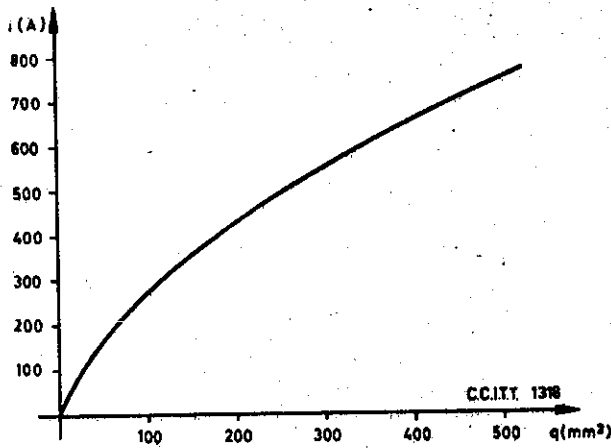
Rys. 4. Normalna obciążalność izolowanych przewodów miedzianych w temperaturze otoczenia 25°C
