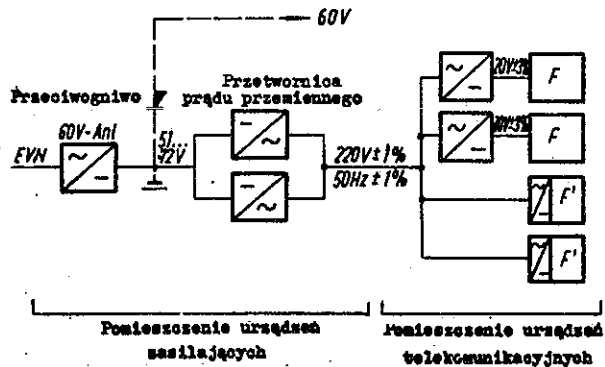
Rys. 3. Zasilania prądem przemiennym
