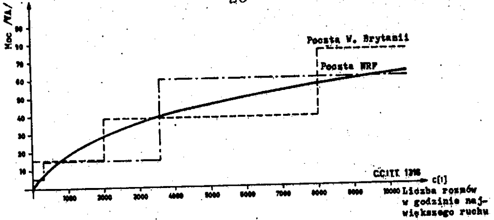
Rys. 3. Typowe wartości poboru mocy prądu dzwonienia i sygnałów akustycznych w funkcji liczby rozmów w godzinie największego ruchu
