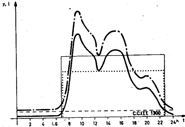
Rys. 1. Charakterystyka ruchu i poboru prądu centrali miejscowej ——— - całkowity pobór prądu ——— natężenie ruchu ..... - średnie natężenie ruchu - - - - stały pobór prądu ——— średni pobór prądu
