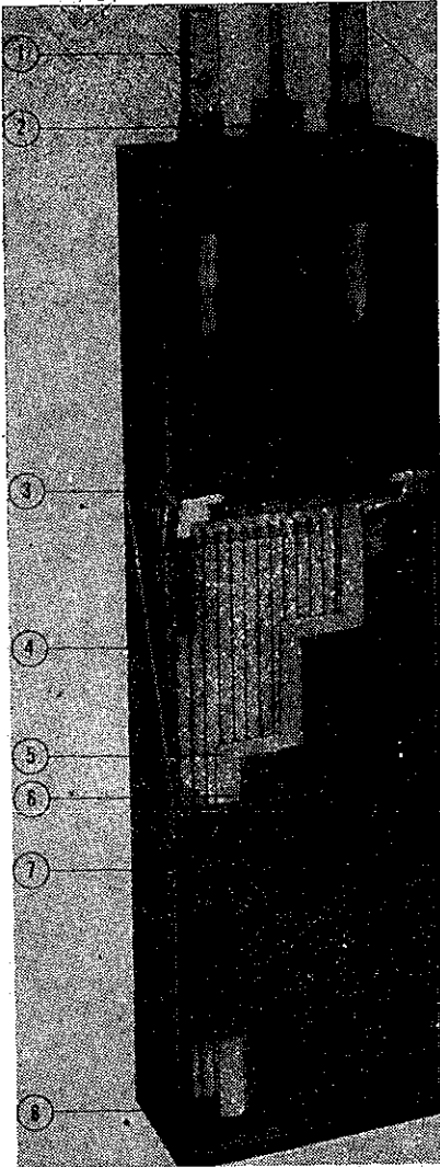
Rys. 1. Akumulator ołowiowy typu zamkniętego z płytami dodatnimi pancernymi (rurkowymi)
