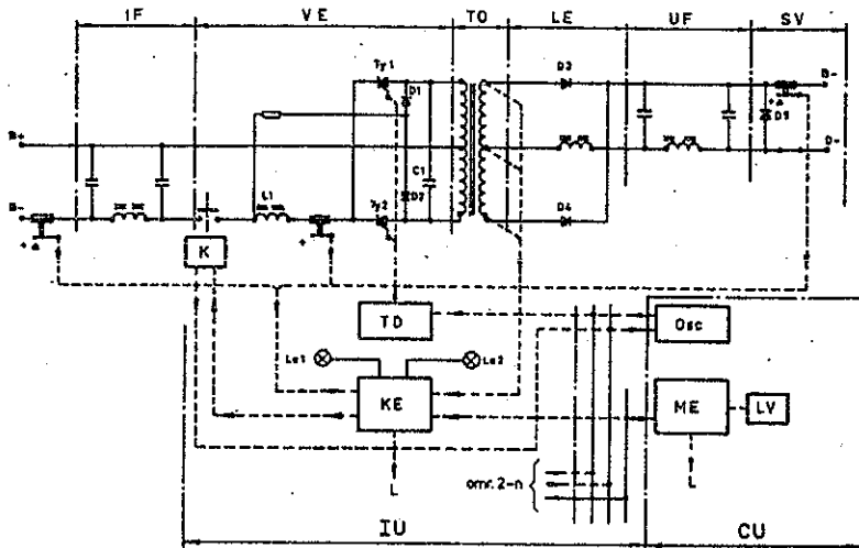
Rys. 8. Uproszczony schemat przetwornicy nieregulowanej 1F - filtr wejściowy, VE - falownik, TO - transformator, LE - prostownik, UF - filtr wyjściowy, SV - zawór obejściowy, K - stycznik, Ty1, Ty2 - tyrystory, D1, D2 - diody komutacyjne, C1, L1 - kondensator i dławik filtru, D3, D4 - diody prostownicze, D5 - dioda obejściowa, TD - zapłonnik, KE - układ kontrolny (monitor), OSC - oscylator 400 Hz, ME - układ rozruchowy (starter), LV - u- kład kontroli napięcia stałego (czujnik), L - alarm, La1 - prze- twornica podczas pracy, La2 - przetwornica nie pracująca, B+, B- bieguny baterii, D - biegun ujemny odbioru, IU - indywidualne wy- posażenie każdej przetwornicy, CU - wyposażenie wspólne (central- ne) przetwornic połączonych równolegle
