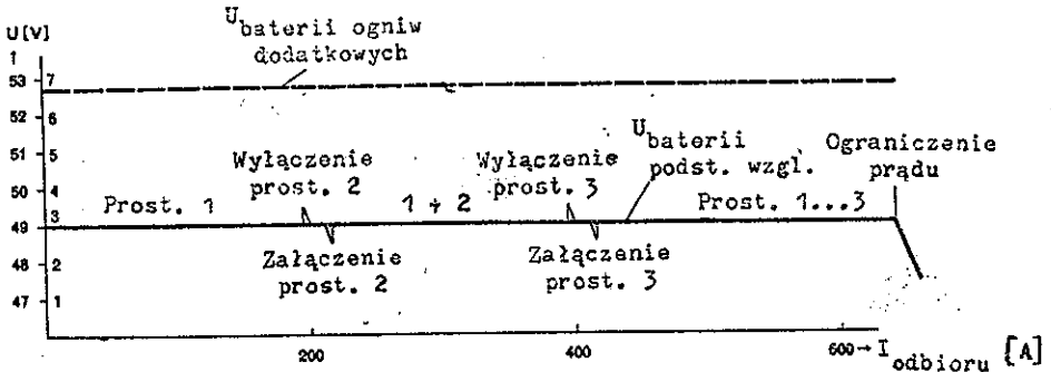
Rys. 4. Przebiegi napięć na zaciskach wyjściowych urządzenia zasilającego typu 600 A z dzieloną baterią i prostownikiem 200 A podczas obecności napięcia w sieci
