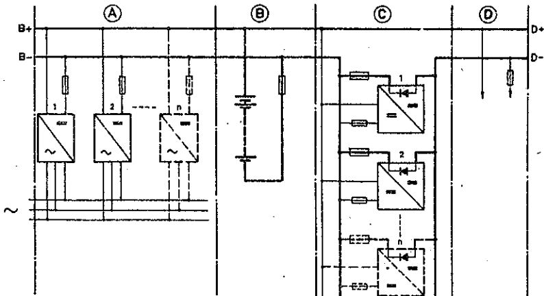
Rys. 6. Schemat blokowy systemu z przetwornicą dodawczą A - prostowniki, B - bateria, C - przetwornice dodawcze, D-od- pływ (odbior), B+,B- - bieguny baterii, D+,D- - bieguny od- bioru
