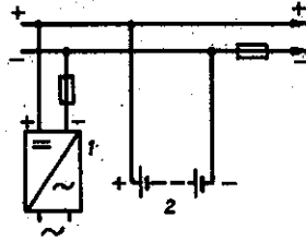
Rys. 2. Schemat blokowy prostego systemu buforowego
