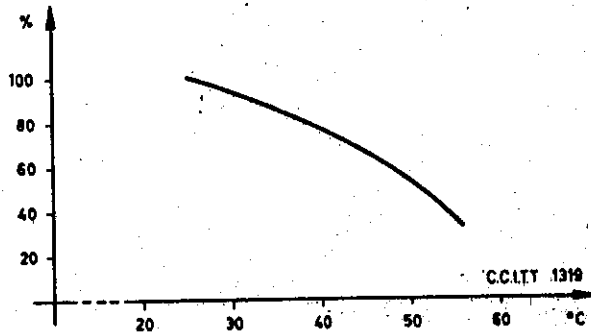
Rys. 5. Zmniejszenie obciążalności izolowanych przewodów miedzianych w zależności od wzrostu temperatury otoczenia powyżej 25°C
