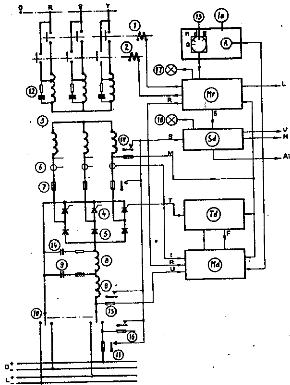
Rys. 5. Schemat blokowy prostownika tyrystorowego 48 V/100 A 1,2 - styczniki, 3 - transformator, 4 - tyrystory, 5 - diody, 6 - przekładnik prądowy, 7 - bezpieczniki o działaniu szybkim, 8 - dławiki filtru, 9 - kondensatory filtru, 10 - łącznik, 11 - bezpiecznik na wyjściu, 12 - zabezpieczenie przepięciowe, 13 - przełącznik pracy: n - praca normalna, d - ładowanie normalne, s - ładowanie szybkie, 14 - zabezpieczenie od przepięć komuta- cyjnych, 15,16 - bezpieczniki układów kontrolnych, 17 - lampka - "ładowanie", 18 - lampka alarmowa - "zanik napięcia" i "stycz- nik wyłączony", 19 - bezpiecznik układu kontroli, Ie - zespół pomiarowy, Mr - zespół przekaźników kontrolnych, SU - zabezpie- czenia, Td - impulsator zapłonowy, Md - zespół czujnikowy, T - impulsy zapłonowe, U - kontrola napięcia, I - kontrola prądu, F - sprzężenie zwrotne, M - zasilanie układów kontrolnych, S - wyłączenie, R - pozioły nastawienia, L - rozkaz podwyższenia napięcia przy ładowaniu automatycznym, AL - alarm uszkodzenia wewnętrznego, N - alarm sieci, V - wyłączenie skutkiem podwyż- szenia napięcia na odbiorze, A - amperomierz
