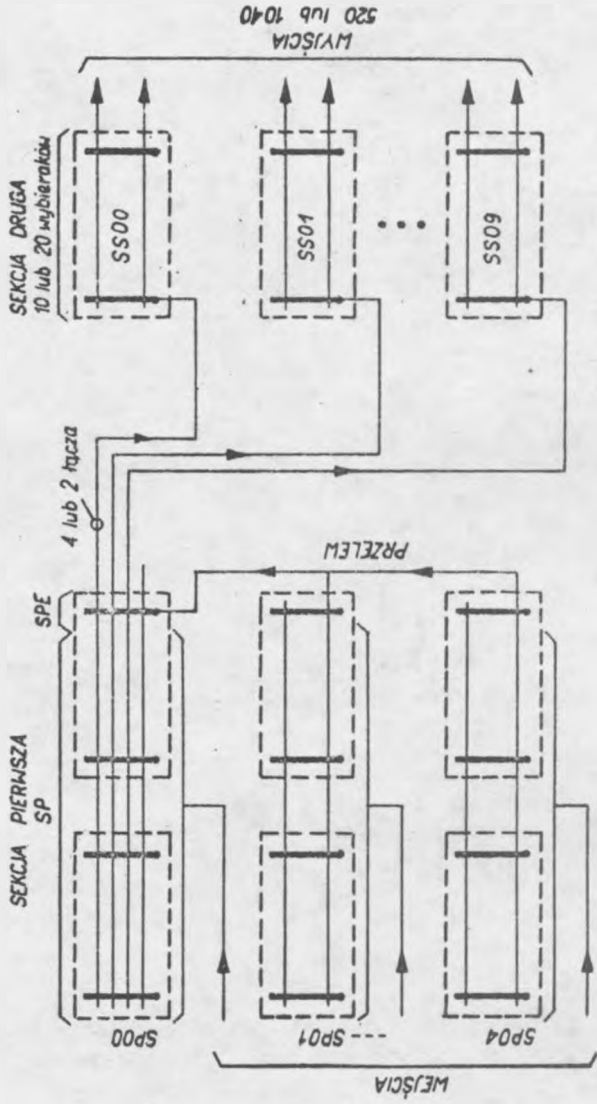
Rys. 5. Ogólna postać struktury bloku grupowego
