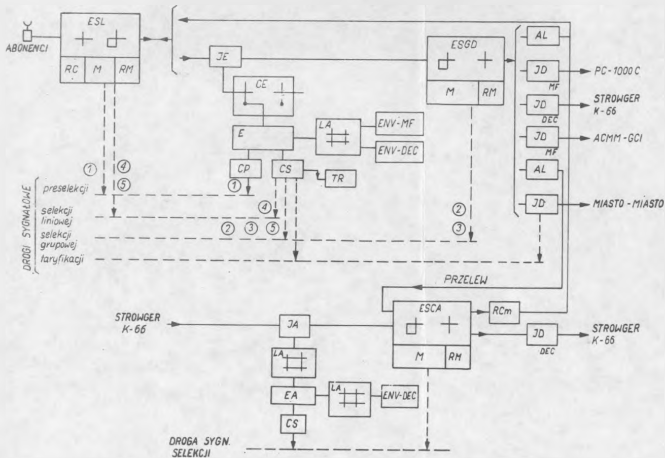
Rys. 8. Schemat obiegu centrali PC-1000C z rozdzielonymi blokami grupowymi, wyjściowym ESGD i przyściowym ESGA
