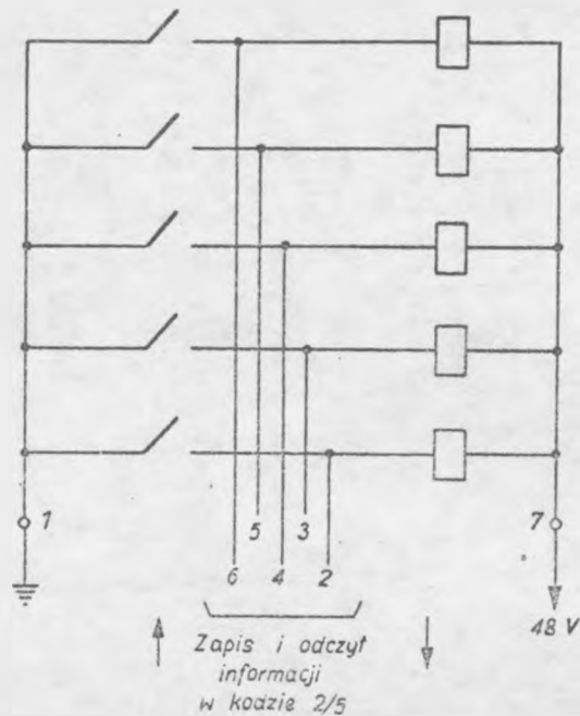
Rys. 10. Schemat wewnętrznych połączeń przełącznika piętkowego
