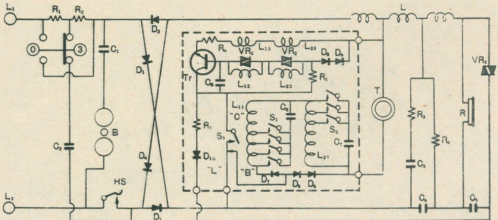
Rys. 4. Schemat aparatu z klawiaturą
