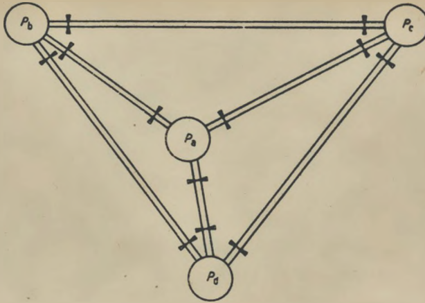
Rys. 6. Model pneumatyczny sieci z synchronizacją wzajemną
