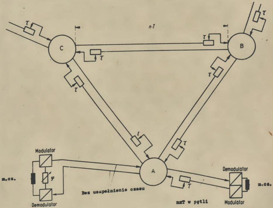
Rys. 7. Zasady wyrównania czasów przeletu / - czas uzupełniającoy, n.T = n.125 \mu s /
