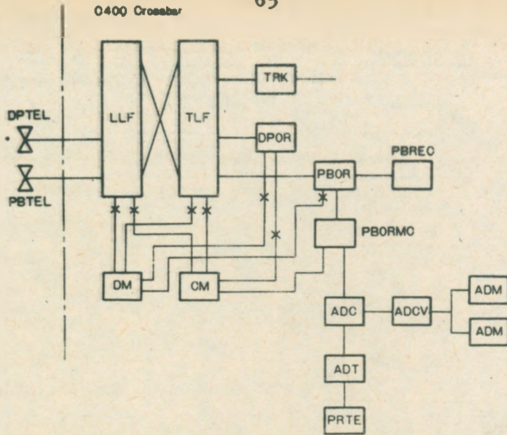
Rys. 1. Schemat blokowy urządzeń systemu telefonicznego z wybieraniem klawiaturą aparatuwą.
