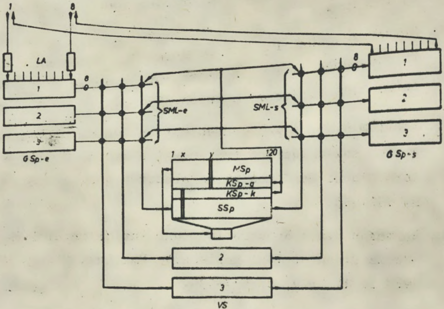
Rys. 5. Sieć kanałów rozmównych przy równoległym układzie komutacji
