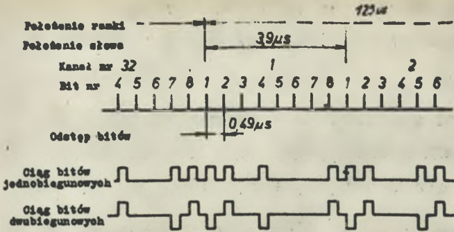
Rys. 1. Sygnał PCM
