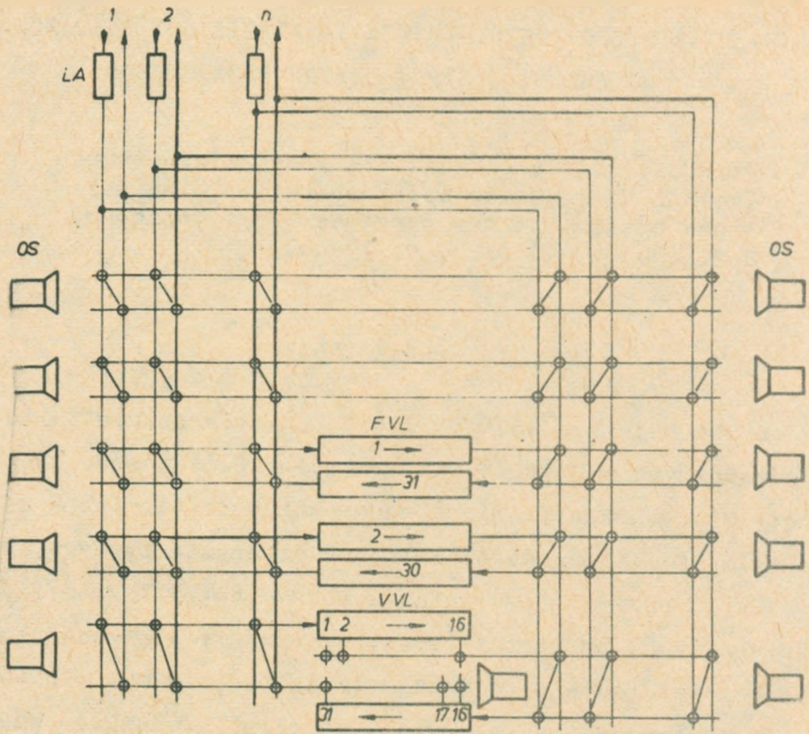
Rys. 3. Sieć kanałów rozmównych przy szeregowym układzie komutacji
