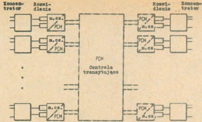
Rys. 4. Sieć zintegrowana z tranzytujuca centrala o komutacji PCM
