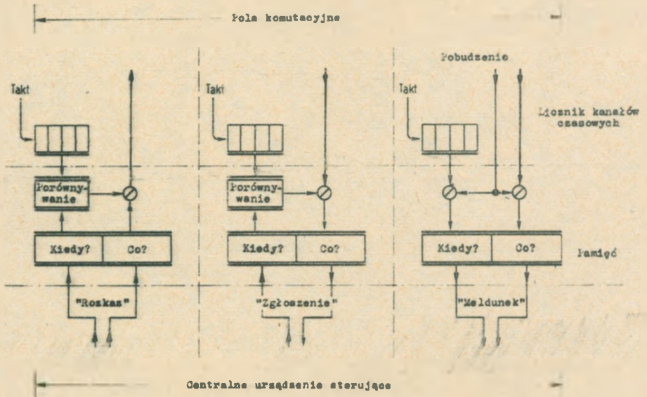
Rys. 11. Przykład dopasowania pola komutacyjnego do procesora
