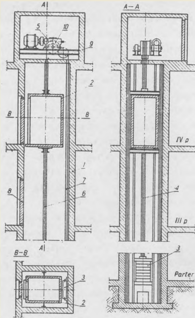
Rys. 14. Układ wyciągu szybowego
