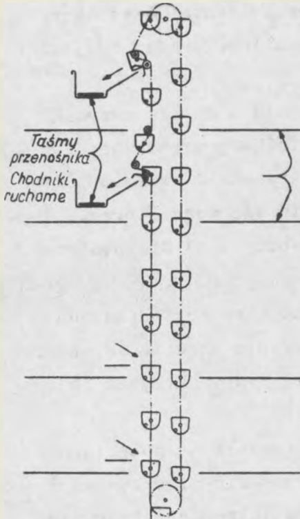
Rys. 2. Schemat działania elewatora kbelkowego z wyładunkiem na dwóch poziomach
