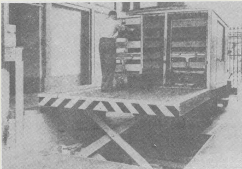
Rys. 13. Platforma załadowcza
