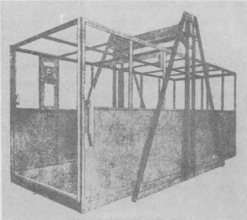
Rys. 15. Kabina nieprzelotowa głęboka wyciągu towarowego osobowego
