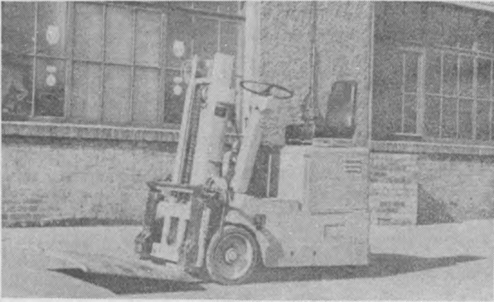
Rys. 12. Wózek jezdniowy podnośnikowy akumulatorowy z opuszczaną platformą załadoczą
