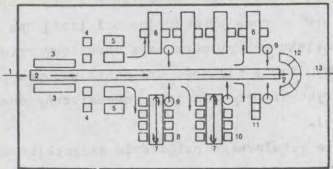
Rys. 24. Schemat przepływu poczty listowej wychodzącej i tranzytowej opracowanej w Upt. Haga
