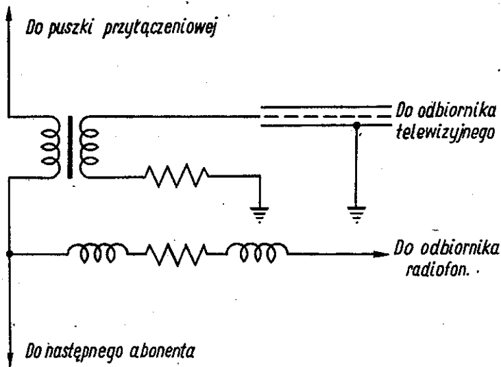
Rys. 3. Układ instalacji u abonenta systemu anteny zbiorowej
