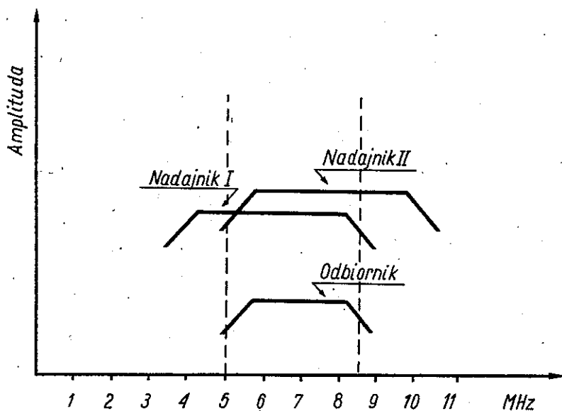
Rys. 10. Układ częstotliwości nośnych "tête-bêche"
