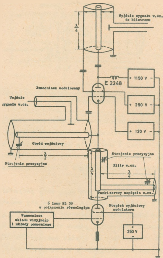
Rys. 14. Schemat wzmacniacza mocy modulowanego sygnałem obrazu
