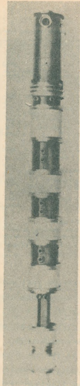
Rys. 5. Klistron typu 4 KM 170000 LA na zakres 300 do 500 MHz /Eitel-McCullough Inc/
