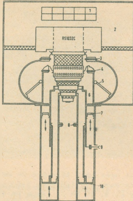
Rys. 17. Widok liniowego wzmacniacza końcowego 2, 4, 10 kW w przekroju
