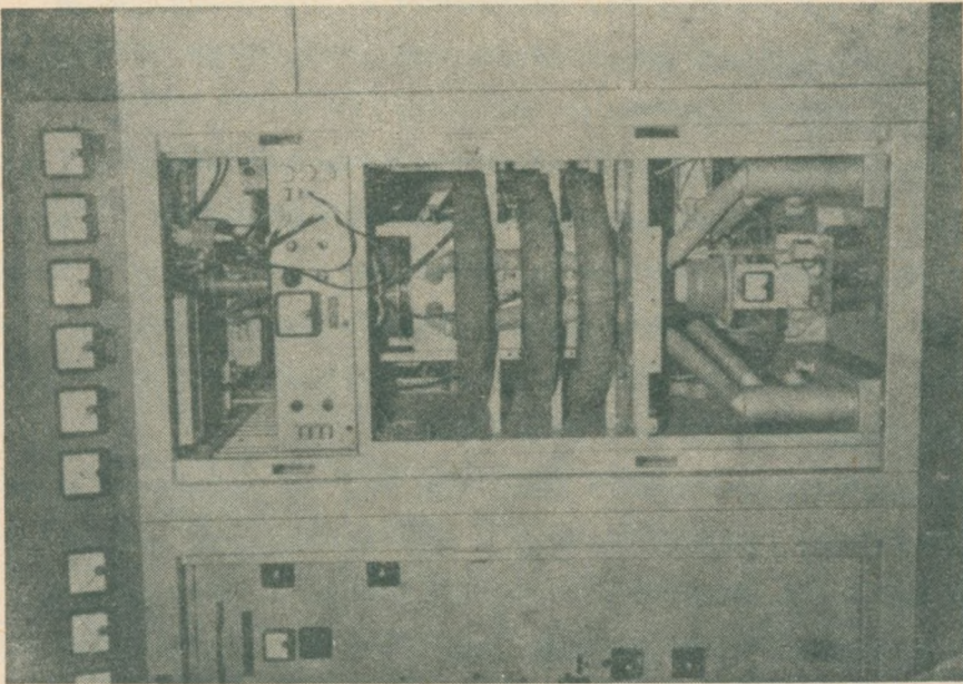
Rys. 7. Klistron trójwójkowy w szafie nadañnika /BBC/
