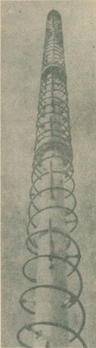
Rys. 20. Antena helikoidalna /BBC/ /długość osiowa przy 654 MHz ok. 4 m/
