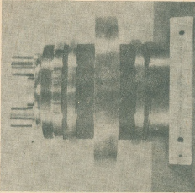
Rys. 4. Wielokatodowa tetroda typu A 2335 C /RCA/ /maks. długość 330 mm, maks. średnica 204 mm/
