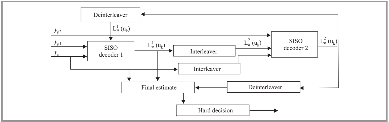
Fig. 2. Turbo decoder.
