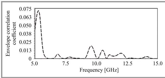
Fig. 12. ECC plot.
