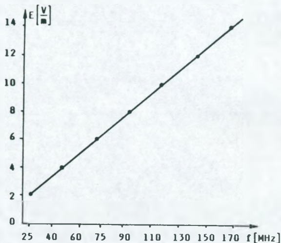
Rys. 8. Natężenie pola elektrycznego w zależności od częstotliwości w zakresie od 25 MHz do 150 MHz dla poziomu zakłócającego 125 dB( \mu\text{V/m} )
