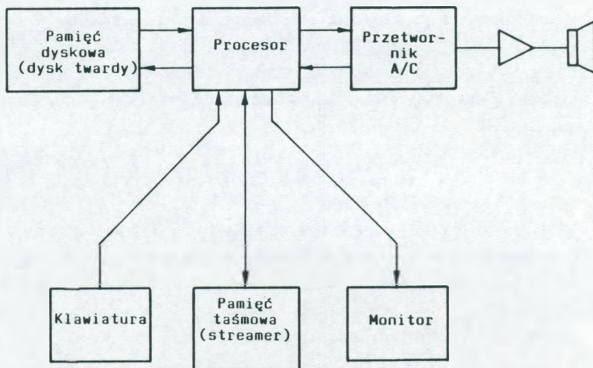
Rys. 4. Budowa bloku odtwarzania sygnałów mowy systemu SDR-1
