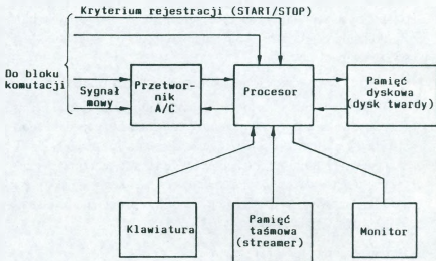
Rys. 3. Budowa bloku rejestracji sygnałów mowy systemu SDR-1
