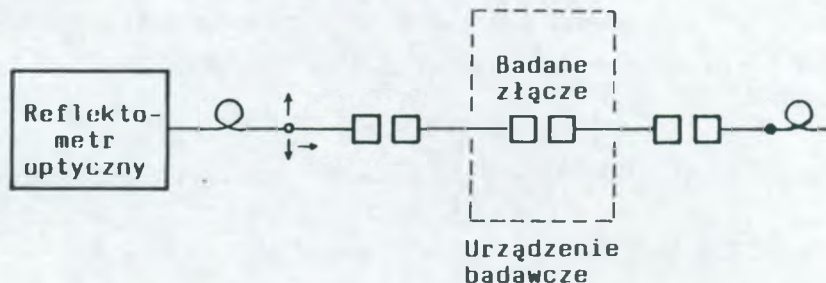
Rys. 2. Schemat zestawu pomiarowego tłumienia złączy optycznych
