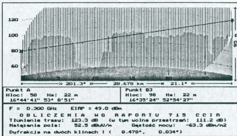
Rys. 8. Profil terenu z analizą propagacją (oryginał jest barwny)
