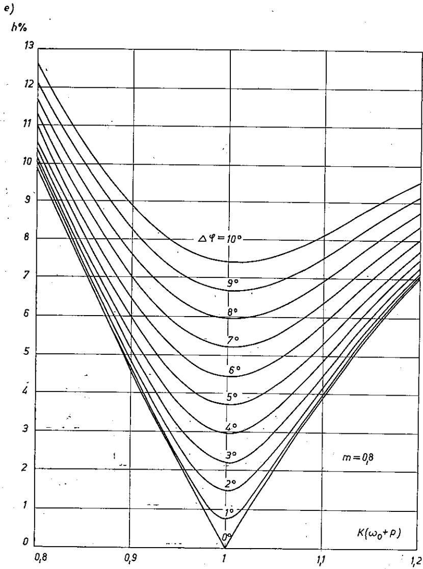
Rys. 5-e) przy m = 0,8 i przy małych wartościach zniekształceń tłumieniowych oraz fazowych.
