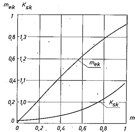
Rys. 1. Zależność wartości zredukowanych współczynników K_{sk} i m_{ek} od rzeczywistej głębokości modulacji amplitudowej sygnału zmodulowanego w systemie CSSB Kahna
