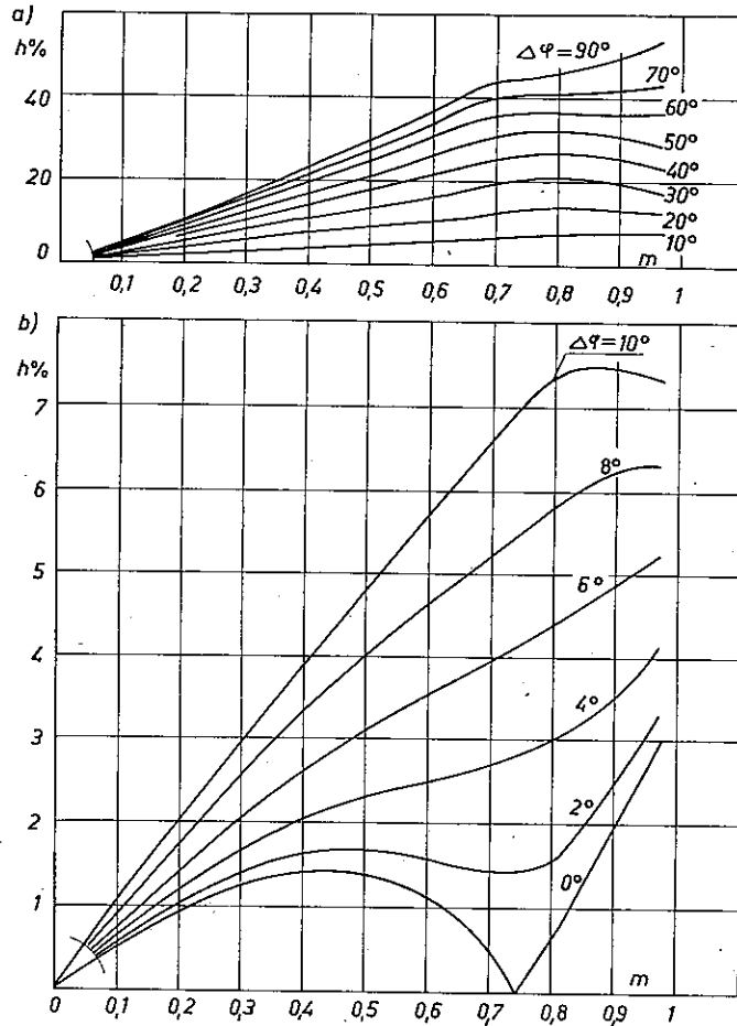
Rys. 10. Zależność zniekształceń harmoniczných obwiedni sygnału zmodulowanego w systemie CSSB – Kahna od głębokości modulacji i przesunięcia fazowego środkowego składnika widmowego
