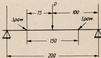
Rys. 6. Pr bka spawana w dw ch miejscach
