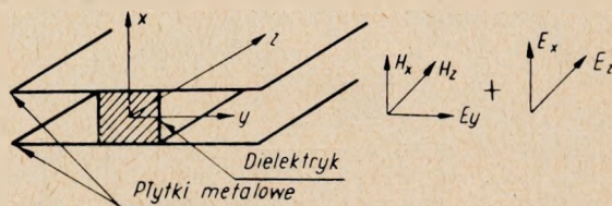
Rys. 11. Falowód Tischer'a
