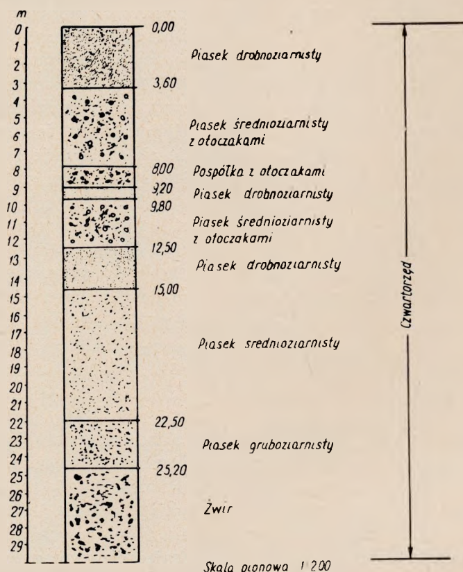
Rys. 2. Profil geologiczny gruntu w miejscu przeprowadzonych badań
