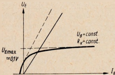
Rys. 7. Dynamiczna charakterystyka obwodu wejściowego wzmacniacza prądu stałego w układzie wspólnego emitera
