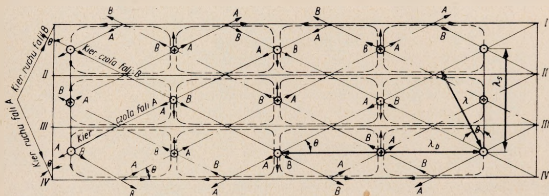
Rys. 1. Powstawanie fal TE w falowodzie jako wynik dwóch płaskich fal elektromagnetycznych A i B
