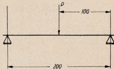
Rys. 7. Pr bka bez spawu
