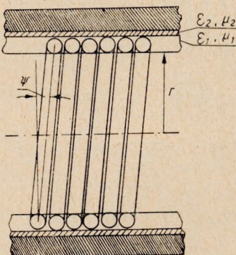
Rys. 19. Falowód zwijkowy
