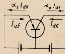
Rys. 3. Prądy tranzystora w przypadku dodatniej polaryzacji emitera i kolektora
