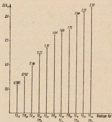
Rys. 15. Stosunek średnicy falowodu D do granicznej długości fali \lambda_0 dla różnych rodzajów fal
