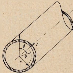
Rys. 5. Falowód o przekroju kołowym
