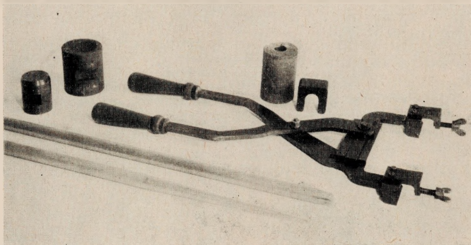
Rys. 8. Kleszcze, tulejka termitowa oraz nasadki używane przy wbijaniu prętów
