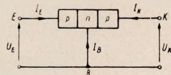
Rys. 2. Tranzystor jako nieliniarny czwórnik elektryczny
