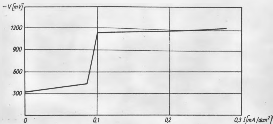
Rys. 3. Katodowa krzywa polaryzacyjna ołowiu w roztworze KCl (1%) zawierającym jony ołowiu
