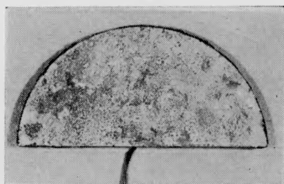
Rys. 11. Wpływ różnych mas aktywujących na charakter zaatakowania płytek magnezowych
