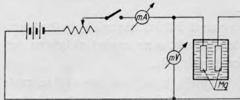
Rys. 9. Zestaw pomiarowy do określenia aktywności mieszanek aktywatora
