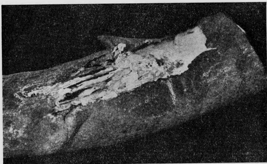
Rys. 5. Kabel TKM 50 \times 4 \times 0,8 ułożony w kanalizacji (tabl. 4)
