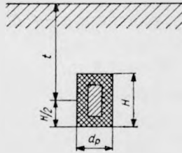
Rys. 14. Protektor osadzony pionowo w ziemi
