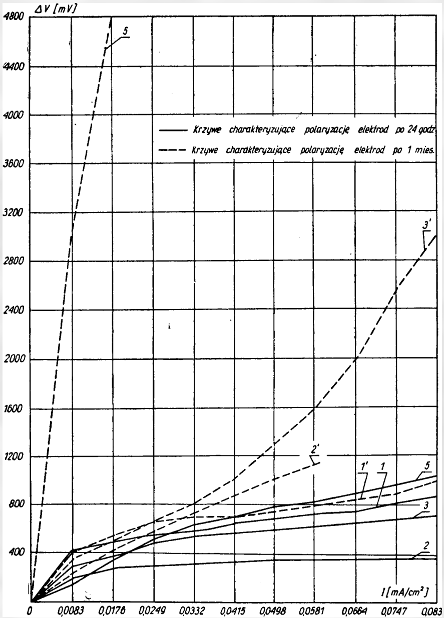
Rys. 10. Wykres zależności zmian potencjałów od gęstości prądu dla elektrod magnezowych w różnych masach aktywujących
