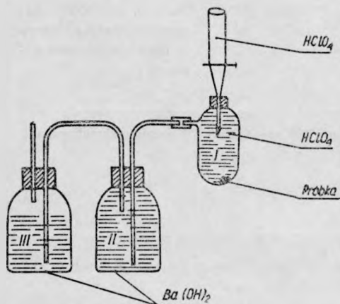
Rys. 1. Aparat używany do pierwszych oznaczeń węglanów
