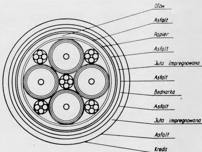
Rys. 15. Kabel TKDWta
