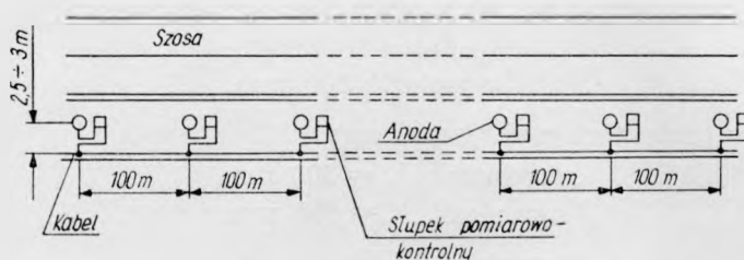
Rys. 16. Schemat ustawienia anod
