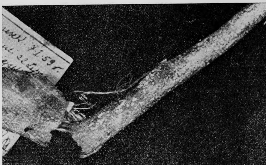
Rys. 6. Kabel TKM 20 \times 2 \times 0,5 ułożony w kanalizacji (tabl. 4)
