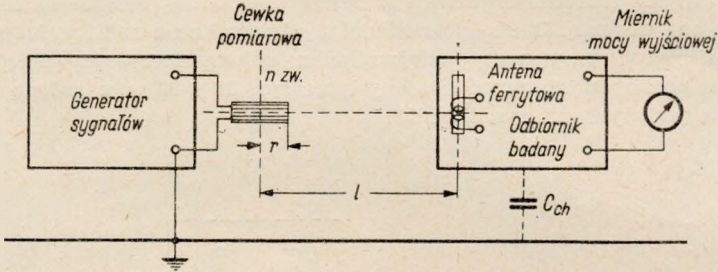
Rys. 32. Układ pomiarowy do badania czułości odbiornika z anteną ferrytową
