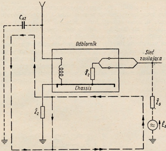
Rys. 6. Rozpływ prądów zakłóceń, przenikających z sieci zasilającej do odbiornika pracującego z anteną otwartą
