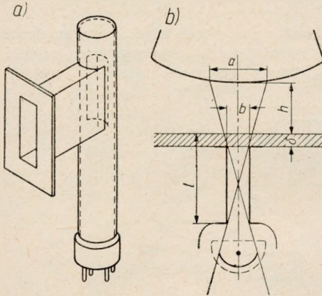
Rys. 3. Sonda fotometru
