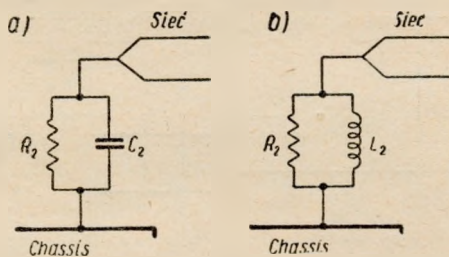
Rys. 3. Układy równoważne zastępujące oporność Z_2 pokazaną na rys. 2
