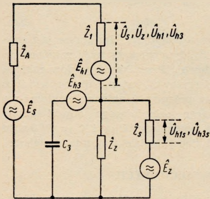
Rys. 11. Uproszczony układ równoważny układowi przedstawionemu na rys. 10
