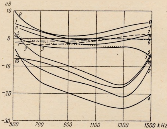
Rys. 28. Porównanie skuteczności filtrów sieciowych, zestawionych na rys. 24, przy przenikaniu zakłóceń z sieci do odbiornika w zakresie fal średnich przy pracy z przerwany przewodem uziemienia
