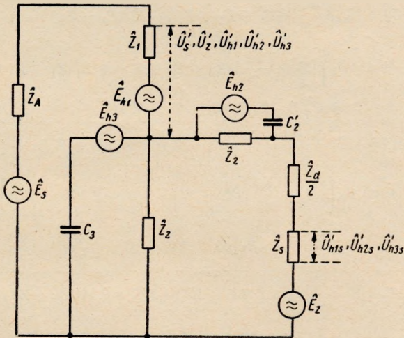
Rys. 13. Uproszczony układ równoważny układowi przedstawionemu na rys. 12
