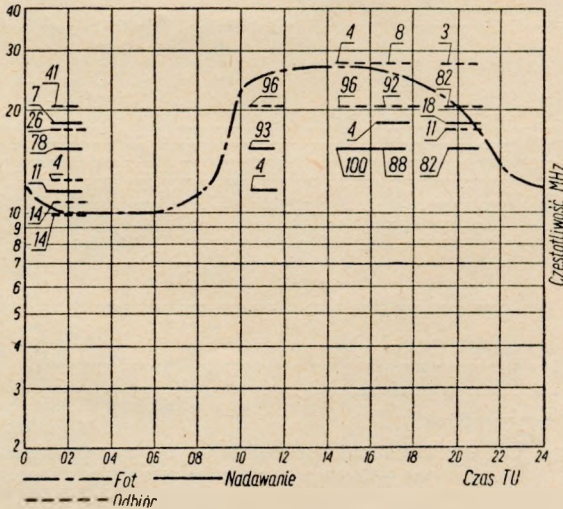
Rys. C1. Współczynniki przechodzenia na trasie Warszawa — Buenos-Aires, marzec 1949
