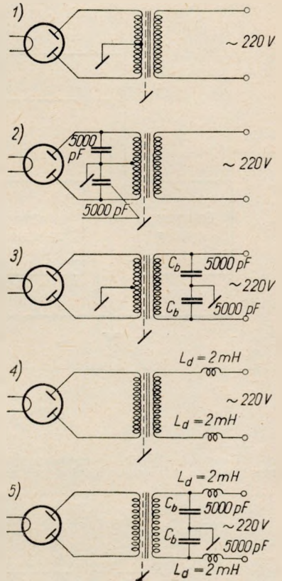
Rys. 21. Układy filtrów sieciowych, zastosowane kolejno przy badaniu odbiornika Mazur
