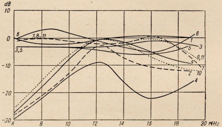
Rys. 29. Porównanie skuteczności filtrów sieciowych, zestawionych na rys. 24, przy przenikaniu zakłóceń z sieci do odbiornika w zakresie fal krótkich przy pracy z krótkim przewodem uziemienia
