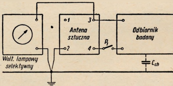
Rys. 14. Układ do pomiaru napięcia o częstotliwości heterodyny, przenikającego do obwodu anteny
