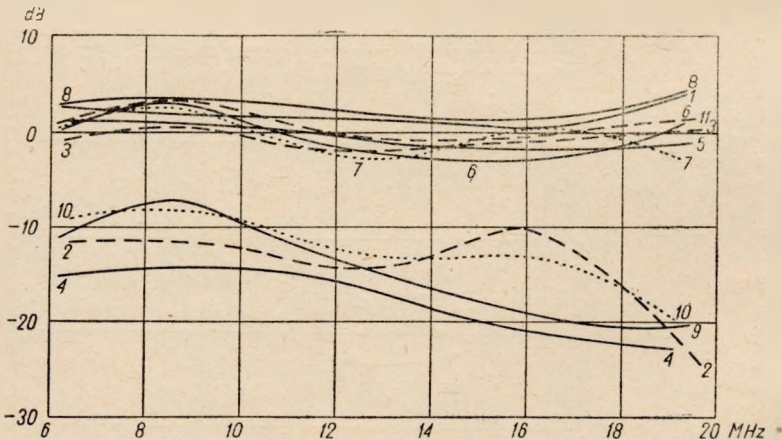
Rys. 30. Porównanie skuteczności filtrów sieciowych, zestawionych na rys. 24, przy przenikaniu zakłóceń z sieci do odbiornika w zakresie fal krótkich przy pracy z przerwany przewodem uziemienia
