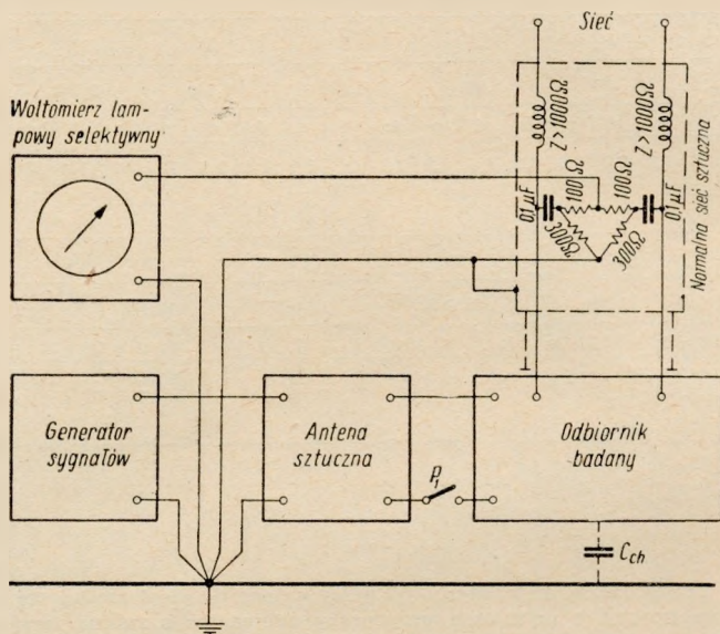
Rys. 20. Układ do pomiaru napięcia o częstotliwości pośredniej, przenikającego do sieci zasilającej
