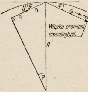
Rys. A2. Warunek wytwarzania wiązki promieni równoległych przez wklęsłe sklepienie
