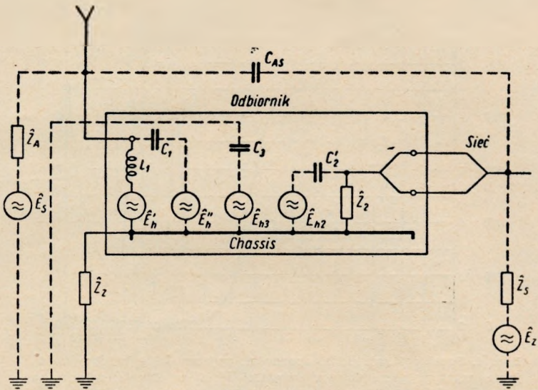
Rys. 2. Siły elektromotoryczne i oporności występujące w urządzeniu odbiorczym
