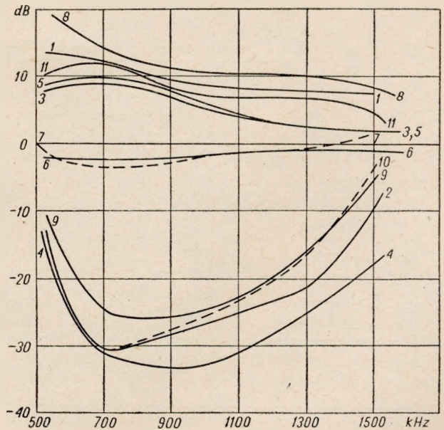
Rys. 27. Porównanie skuteczności filtrów sieciowych, zestawionych na rys. 24, przy przenikaniu zakłóceń z sieci do odbiornika w zakresie fal średnich przy pracy z krótkim przewodem uziemienia
