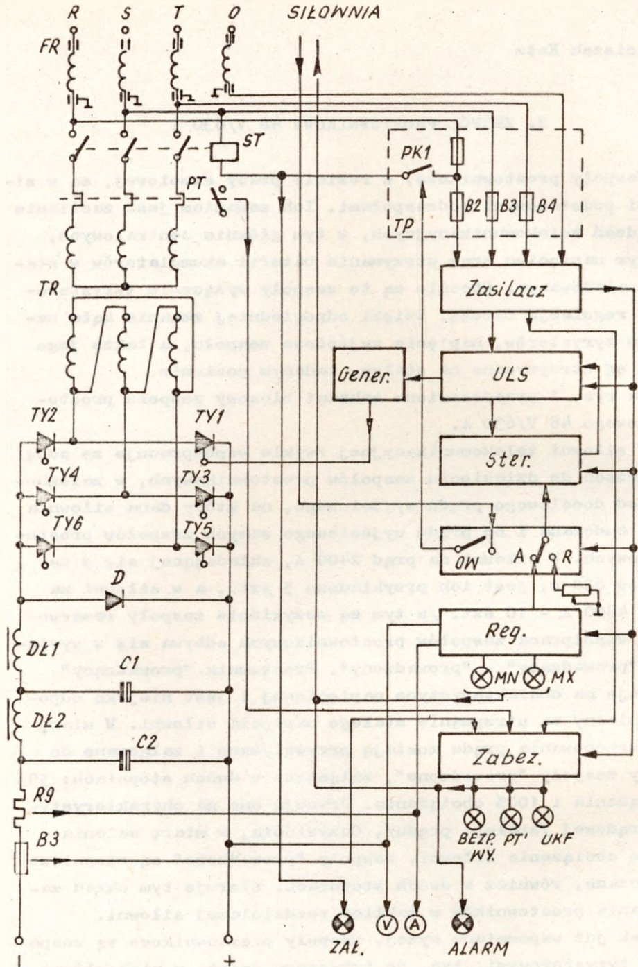
Rys. 1. Schemat blokowy zespołu prostownikowego 48 V/630 A
