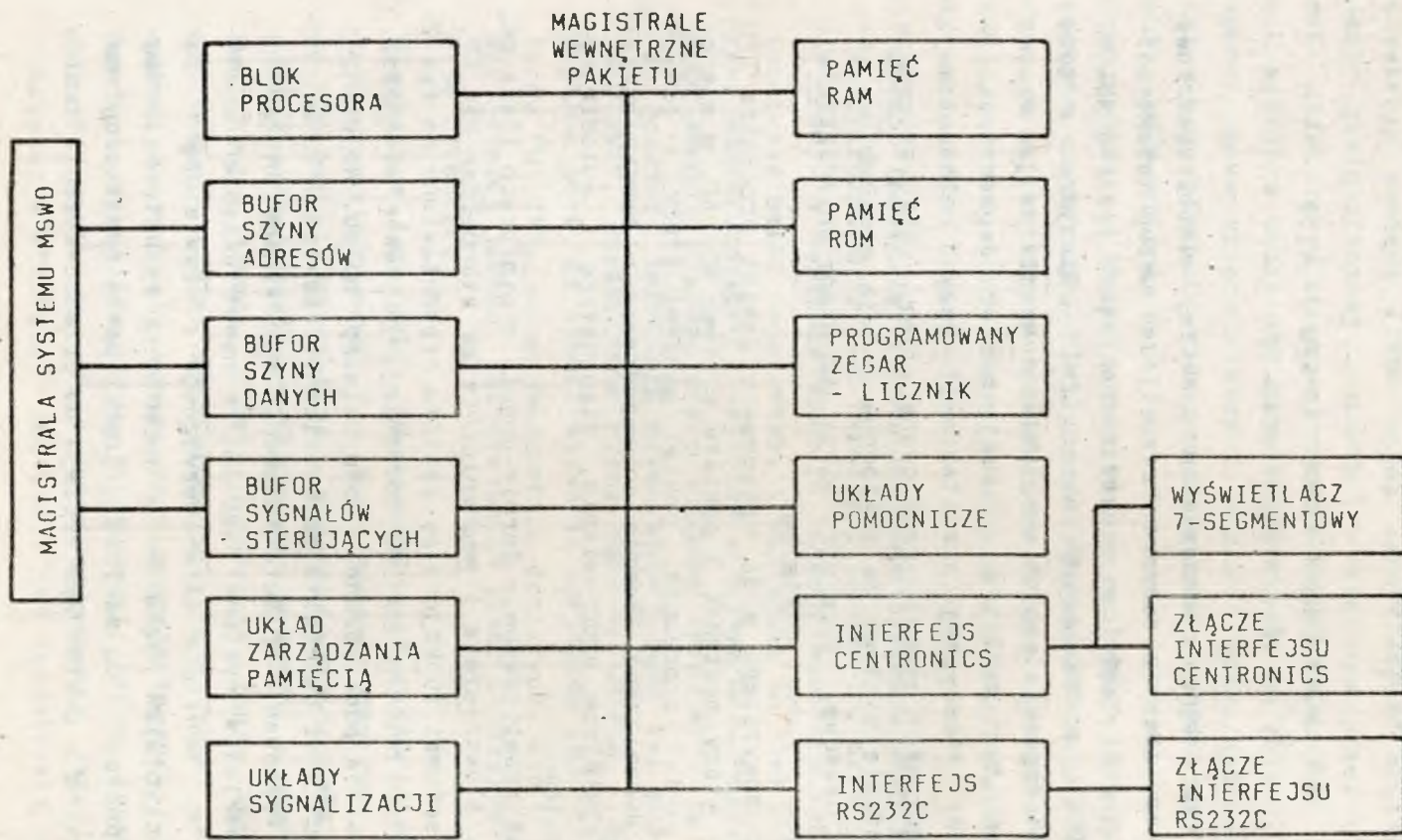
Rys. 2. Blokowy schemat funkcjonalny pakietu
